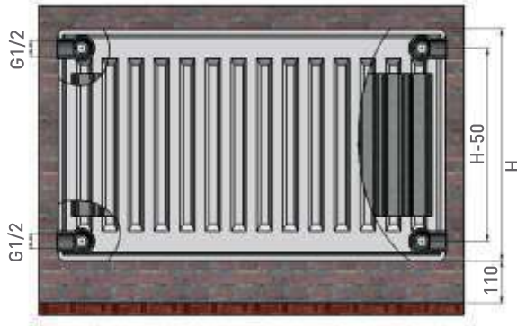
Termolux Klasik Ön Kesit Görünümü
